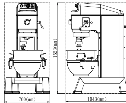
(SP-A62H/SP-B62H) DIMENSION
